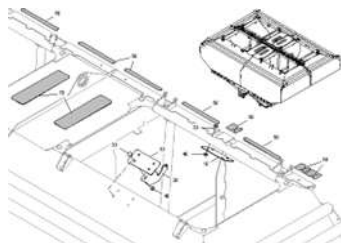
ЕТВ-0000007796, Бак 13000 л, Навесное оборудование (с 01.2015)
