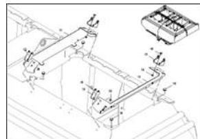
ЕТВ-0000007842, Задняя часть 13000 л, рамная часть (2) (с 01.2015)
