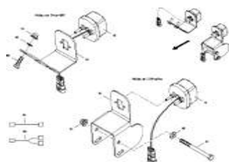
ETB-0000008118, Schlussleuchte Schnecke/Greengrill
