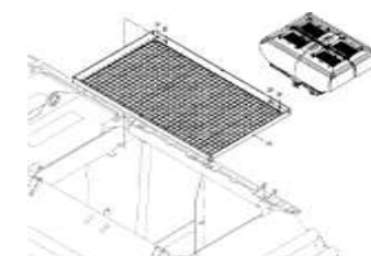
ЕТВ-0000007798, Бак 1300 л, решетчатая решетка
