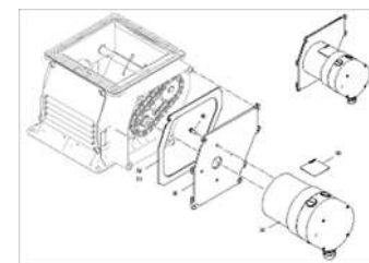
ЕТВ-0000007182, Подмножество электроприводов
