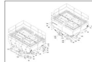
ЕТВ-0000006742, Задняя часть 1300 л фойлинг (с 01.2015)
