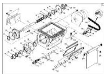
ЕТВ-0000003276, Одинарный дозатор прав.
