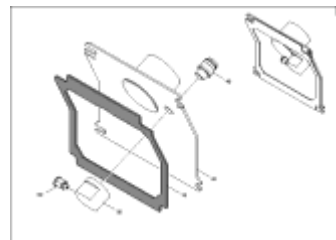
ЕТВ-0000003278, Комплект деталей для системы подачи под давлением
