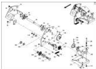
ЕТВ-0000003237, Привод Primera DMC 12001 перед (2)
