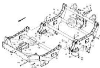
ЕТВ-0000007821, Задняя часть 13000 л, рамная часть спереди/сзади (с 01.2015)
