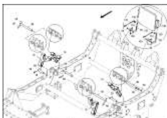
ЕТВ-0000007842, Задняя часть 13000 л, рамная часть (2) (с 01.2015)
