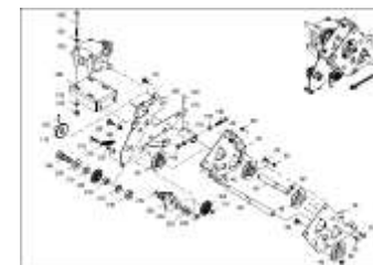
ЕТВ-0000003238, Привод Primera DMC 12001 перед (3)
