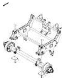
ЕТВ-0000003229, Тормозная ось со стояночным тормозом для задней части 13000 л (2)
