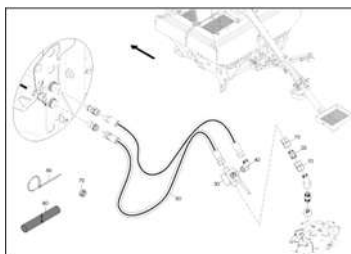
ЕТВ-0000003338, Загрузочный шнек 13000L VM (9) / дополнительный пакет привод ВКН
