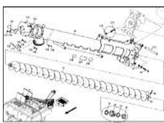
ETB-0000003331, Загрузочный шнек 13000L VM (2) / подающая труба выпуск
