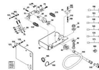
ЕТВ-0000003267, Монтажный комплект SLUE Isobus 13000 L предв. смонт.
