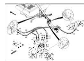
ETB-0000003336, Загрузочный шнек 13000L VM (7) / гидр. Блок управления
