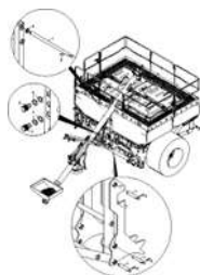
ЕТВ-0000003339, Загрузочный шнек для задней части 13000 л (1)
