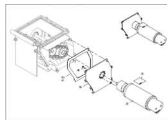
ЕТВ-0000007180, Подмножество электроприводов
