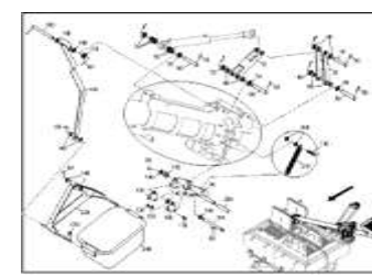
ETB-0000003333, Загрузочный шнек 13000L VM (4) / монтажные детали впускная/выпускная труба
