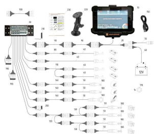
ЕТВ-6000000131 66500339 Система контроля высева СКИФ-28 до 07.2025
