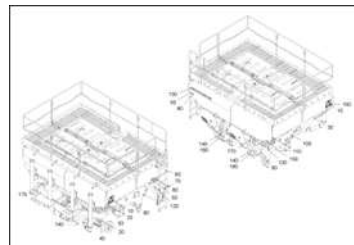
ЕТВ-0000006742, Задняя часть 1300 л фойлинг (с 01.2015)
