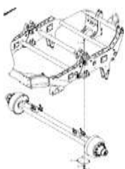
ЕТВ-0000003230, Оси (1)
