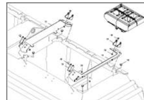
ЕТВ-0000007878, Задняя часть 13000 л, накладные детали (с 01.2015)
