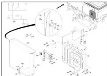
ЕТВ-0000003371, Оборудование машины DMC 13000L Isobus предв. смонт. (3) / электроблок, отдельные детали
