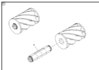
ETB-0000009128, Дозирующий ролик 700 куб.см
