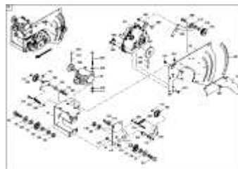
ЕТВ-0000003711, Узел редуктора удобрения лев. 12001
