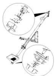
ЕТВ-0000003343, Загрузочный шнек для задней части 13000 л (5)
