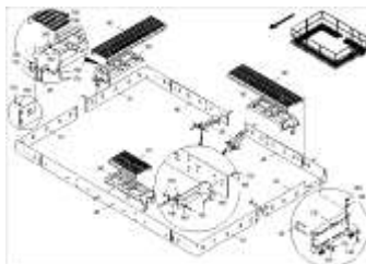
ЕТВ-0000003227, Лестница и группа платформы (3)
