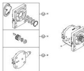
ЕТВ-0000009547, Гидравлический двигатель GF048
