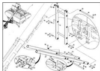
ETB-0000003334, Заправочный шнек: 13000 л (5) / Motageteile Schütze
