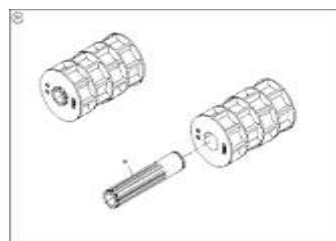
ЕТВ-0000008387, Дозирующий ролик 350 см³
