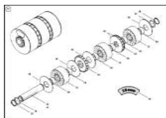
ЕТВ-0000007912, Дозирующий ролик 20 см³
