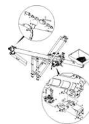
ЕТВ-0000003344, Загрузочный шнек для задней части 13000 л (6)
