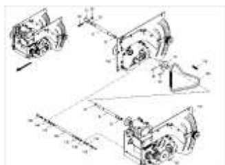
ЕТВ-0000003709, Привод семена удобрения лев.
