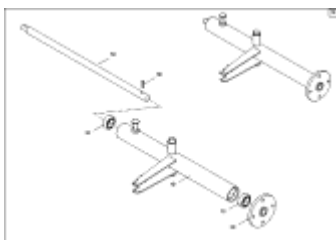
ЕТВ-0000008032, Маятник
