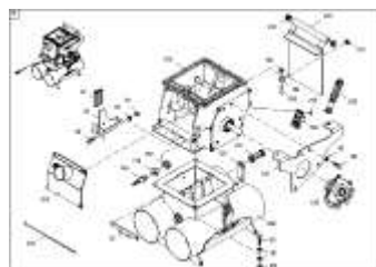
ЕТВ-0000005572, Дозатор 13000L слева, механический
