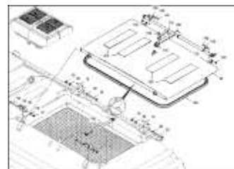
ЕТВ-0000007862, Контейнер 13000 л , крышка под давлением (01.2015-07.2023)
