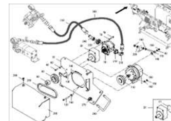
ETB-0000007461, Генератор переменного тока , Бортовое электропитание
