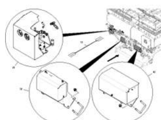
ETB-0000003259, Бортовое электропитание DMC 13000L
